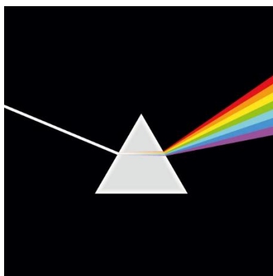
Figura 1: Prisma decompondo a luz
