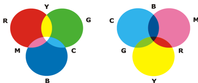
Figura 3: Cores aditivas e subtrativas
